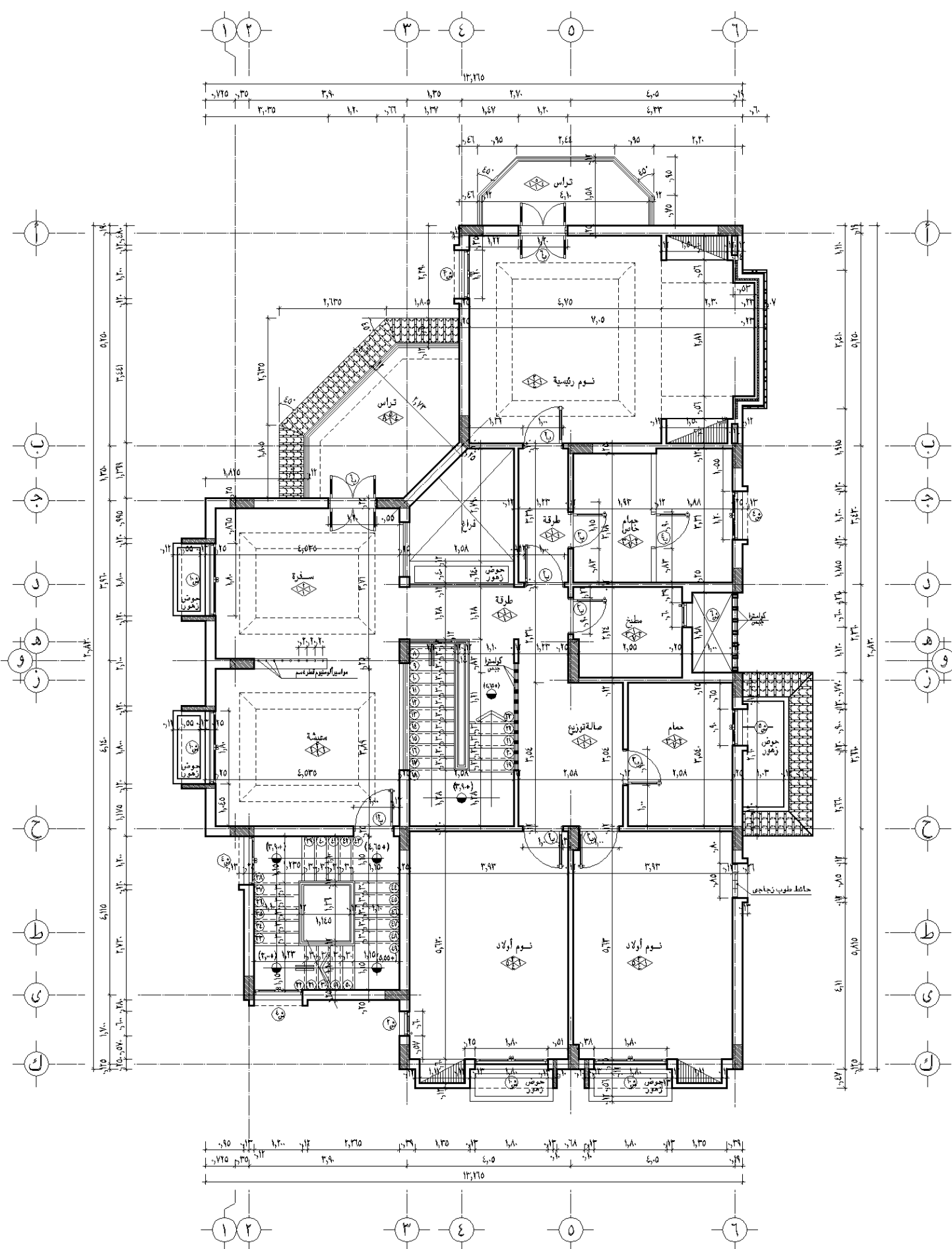
المسقط الأفقي للدور الأول علوي ١ / ٥
