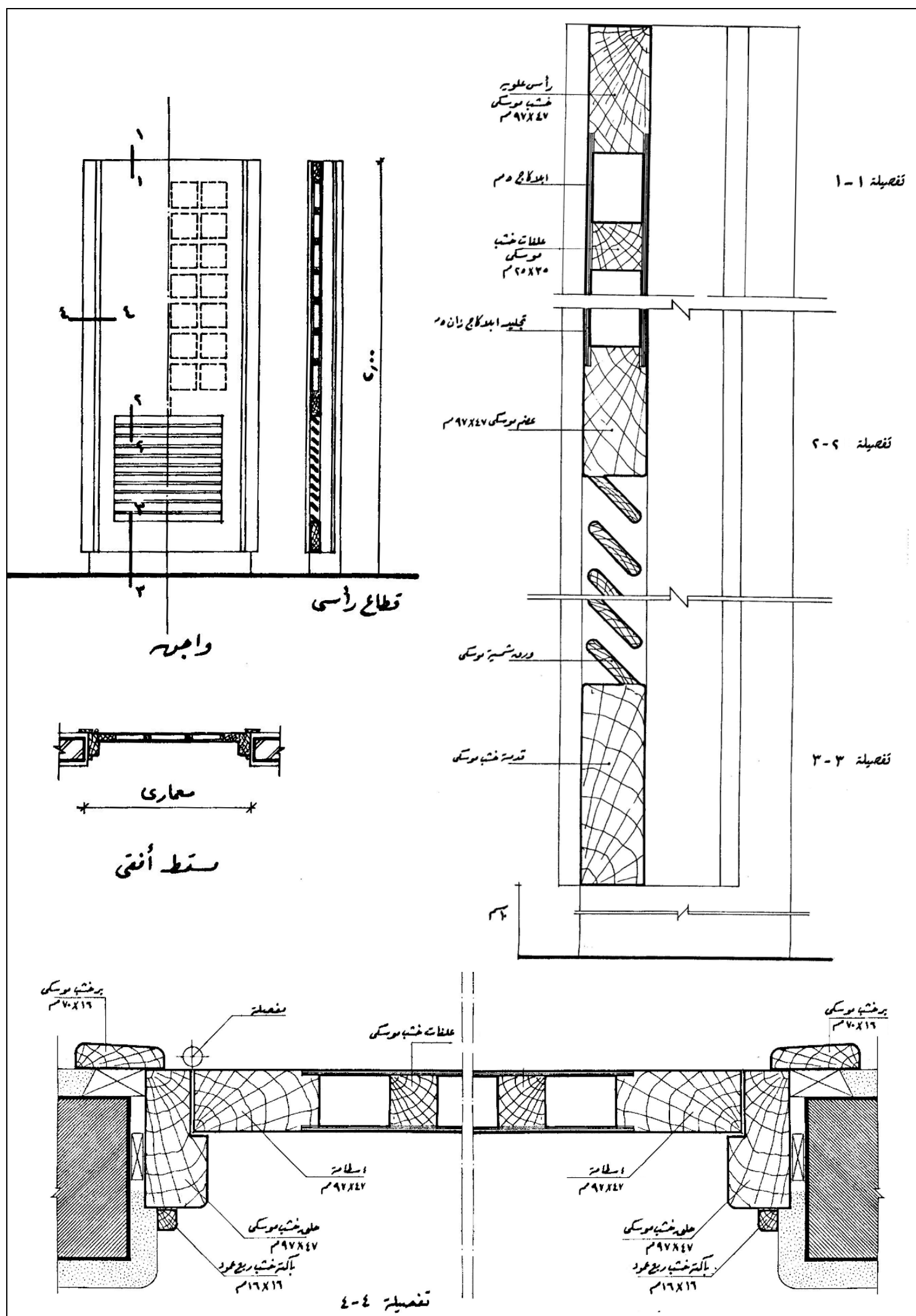
شكل رقم (٥٣) : مثال على باب تجليد أبلجاج بشمسية من أسفل.
