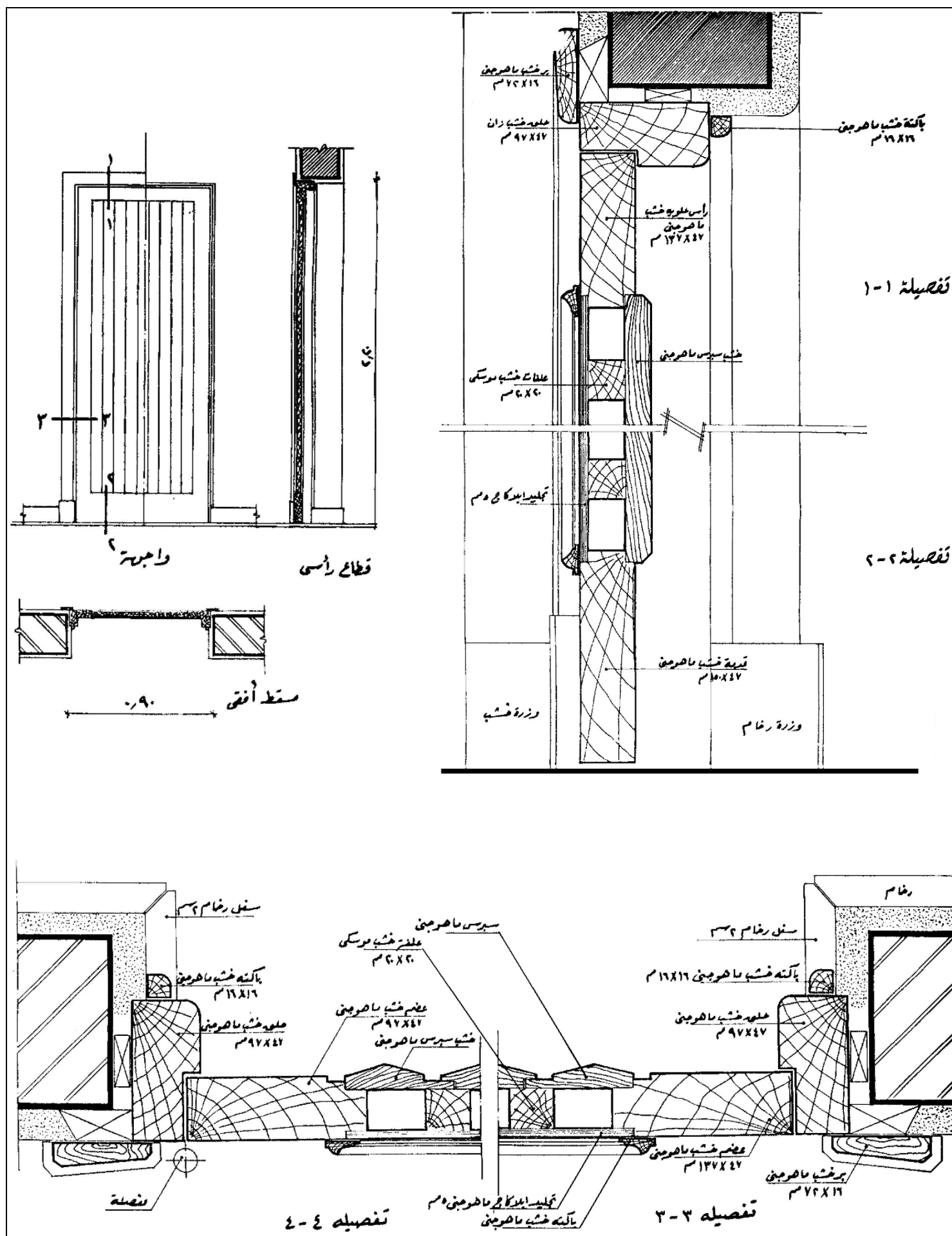
شكل رقم (٥٤) : مثال على باب تجليد أبلجاج من الداخل وتجليد سبرس من الخارج.
