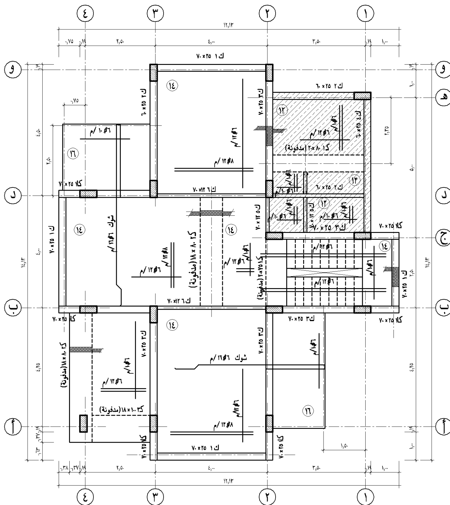
شكل رقم (٣١) نموذج توضيحي لشكل المسقط الأفقي الإنشائي للأسقف والكمرات.
